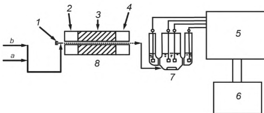
1 — мембрана для ввода пробы; 2 — вход; 3 — зона окислительного горения; 4 — выход; 5 — микрокулометр; 6 — потенциометрический самописец; 7 — ячейка для титрования; 8 — пиролизная печь; а — кислород, O_2 ; b — газ-носитель
