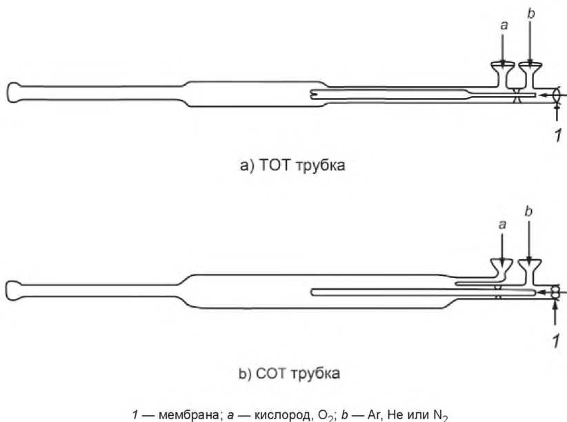
Рисунок 2 — Типовые конструкции трубок для сжигания
