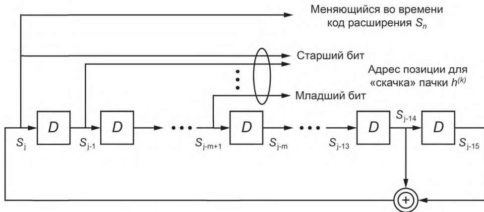
Рисунок 11 — Реализация скремблера в виде РСЛОС
