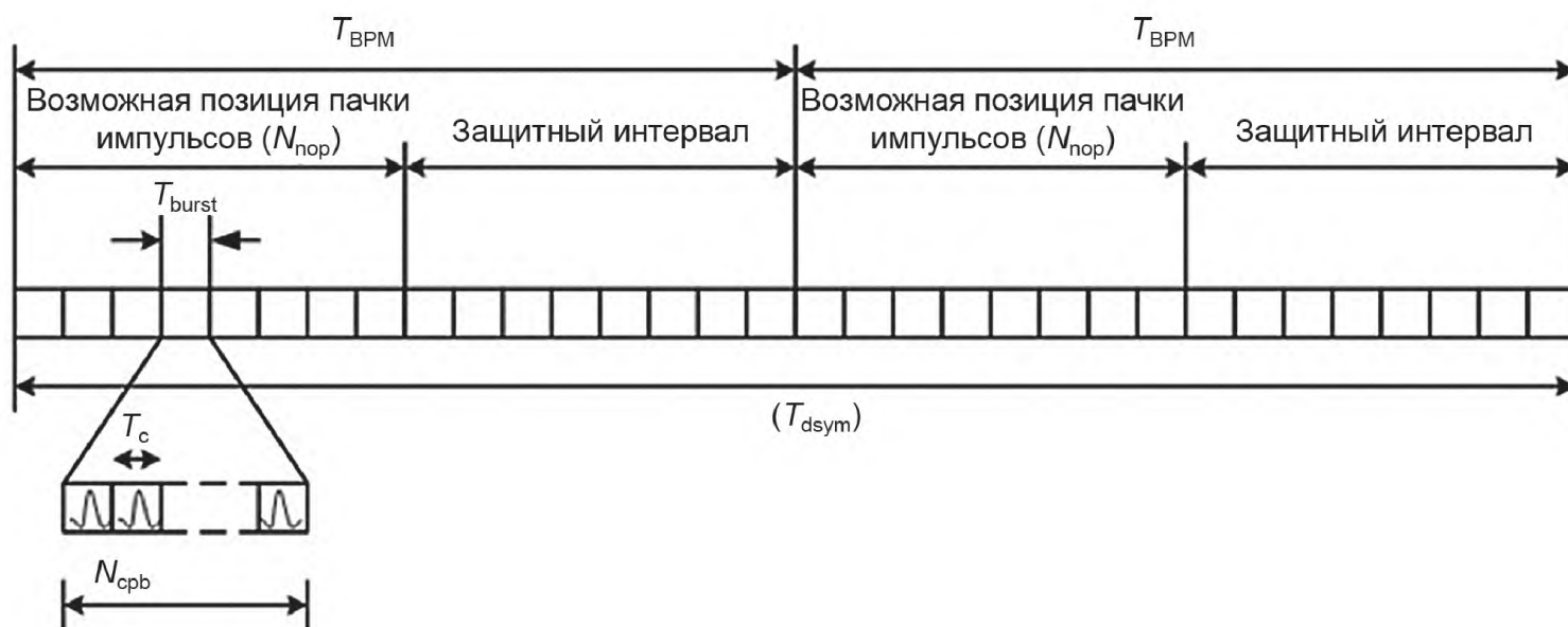
Рисунок 5 — Структура символа
