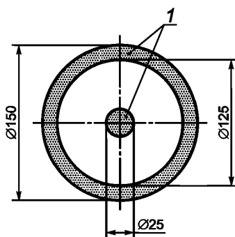
1 — контактное вещество (4.2.5)
