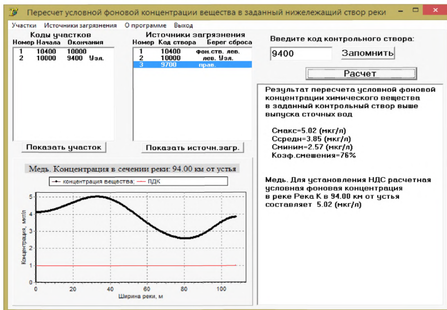
Рисунок Г.17 – Вид экранной формы представления результата перерасчета условной фоновой концентрации меди в створ G реки К
