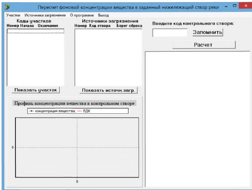
Рисунок Б.1 - Главная экранная форма программы
