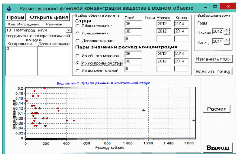
Рисунок Г.3 – Зависимость изменения содержания нефтепродуктов от расхода воды в створе G реки В
