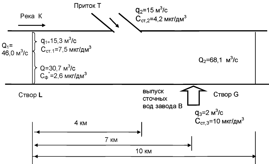
Рисунок Г.11 – Схема рассматриваемого участка реки К
