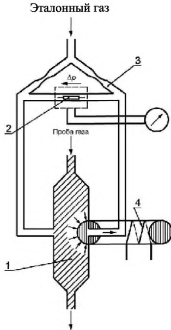
1 — камера измерений; 2 — микродатчик расхода; 3 — капилляры; 4 — электромагнит
