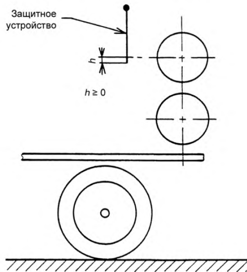
Рисунок 1 – Защитное устройство
