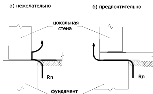
Рисунок 2 – Нерекомендуемое и рекомендуемое решения узла сопряжения плиты пола с фундаментом
