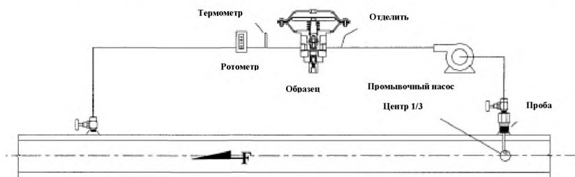
Рисунок 4 -Типичная установка образца для насоса
