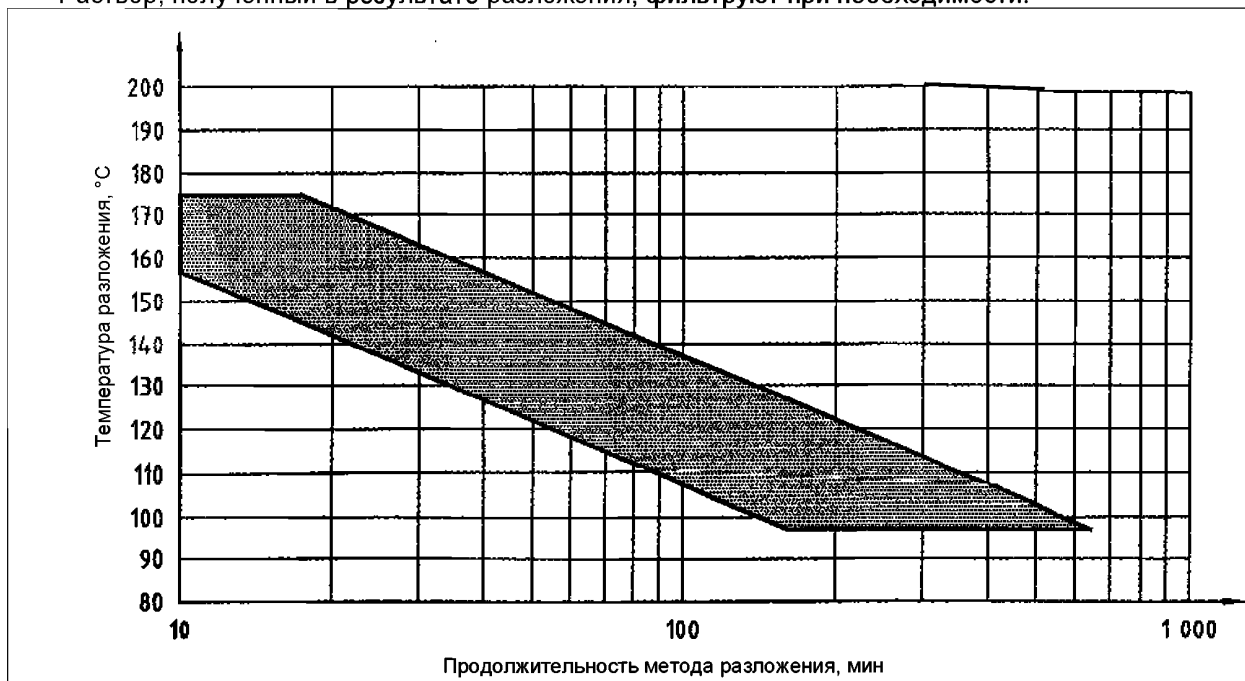
Рисунок 1 – Диапазон разрешенных температур и продолжительности метода разложения
