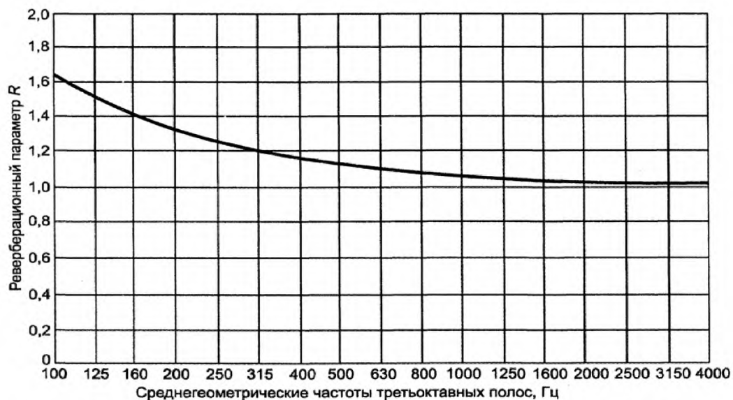
Рисунок Б.3 – Значение реверберационного параметра R для камеры объемом 70 \text{ м}^3 в функции среднегеометрической частоты третьоктавной полосы
