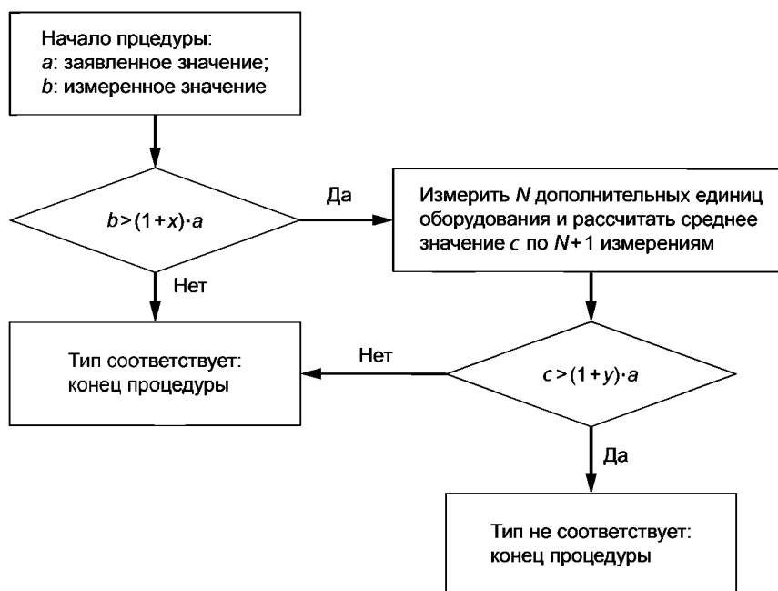
Рисунок А.1 — Алгоритм процедуры верификации
