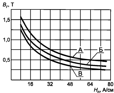
Рисунок 2 — График определения способа контроля по остаточной индукции и коэрцитивной силе металла
