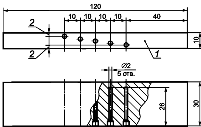
1 — брусок; 2 — цилиндрическое отверстие, закрытое винтом М 2,5
