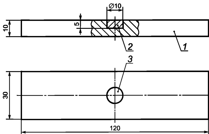
1 — брусок; 2 — вставка с несплошностью; 3 — подповерхностная несплошность
