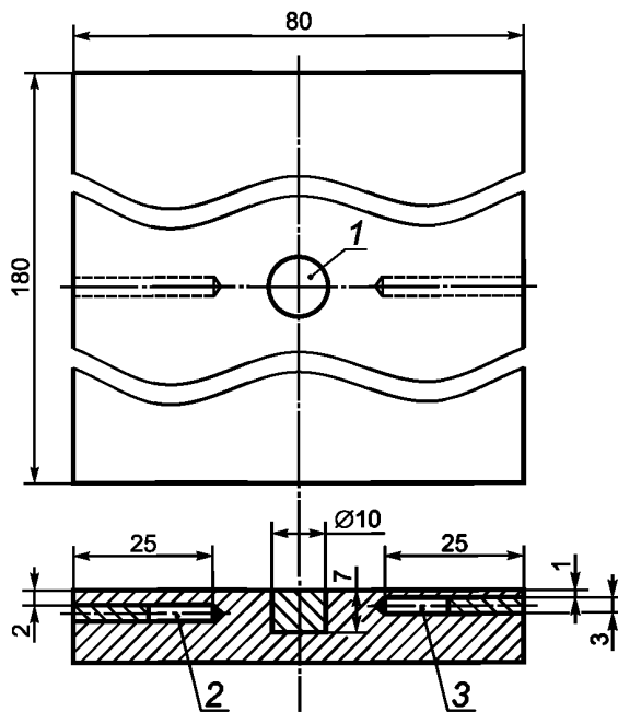
1 — вставка с несплошностью; 2, 3 — подповерхностные несплошности
