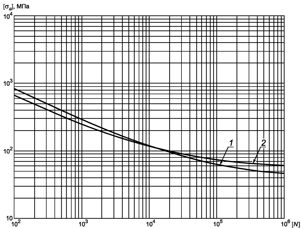
1 — М2, М3, МЗр при A = 0,39 \cdot 10^5 МПа, B = 76,5 МПа, T = 250 °С; 2 — ЛС59-1-1, Л63, ЛО62-1, ЛЖМц при A = 0,3 \cdot 10^5 МПа, B = 108,8 МПа, T = 250 °С
