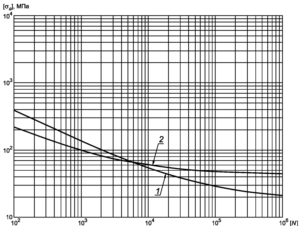
1 — AMцС, AMг2, AMг3 при A = 0,18 \cdot 10^5 МПа, B = 34 МПа, T = 150 °С; 2 — AMг5, AMг6 при A = 0,86 \cdot 10^4 МПа, B = 84 МПа, T = 150 °С
