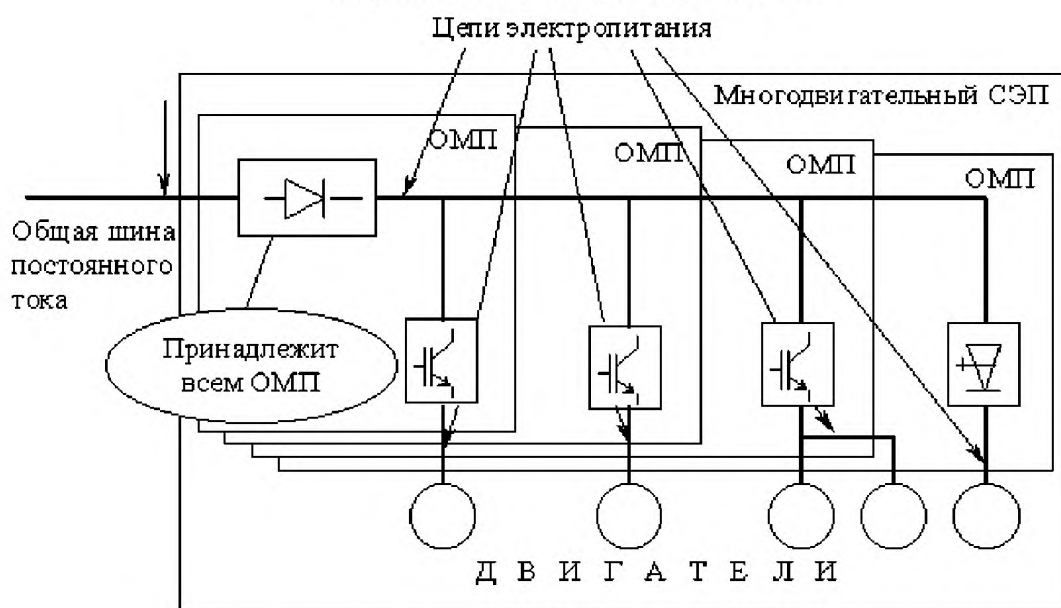
Рисунок 3 – Цепи электропитания СЭП с общей шиной постоянного тока
