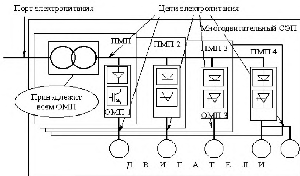
Рисунок 4 – Цепи электропитания СЭП с общим входным трансформатором
