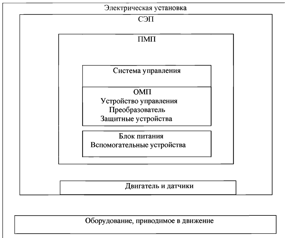
Рисунок 1 - Составные части электрической установки, включающей СЭП
