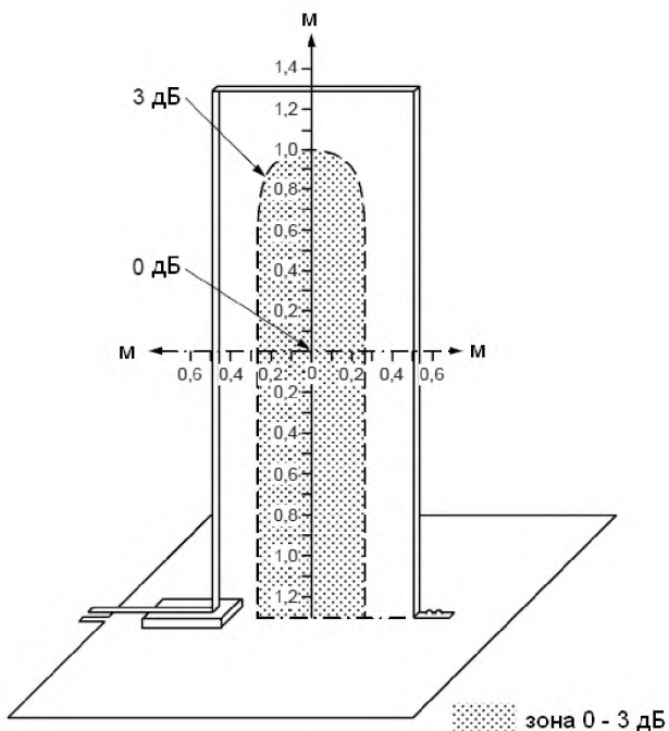
Рисунок В.7 – Зона \pm 3 дБ магнитного поля, создаваемого индукционной катушкой прямоугольной формы (с размерами сторон 1 × 2,6 м) в плоскости катушки (нижней стороной индукционной катушки является эталонная пластина заземления)
