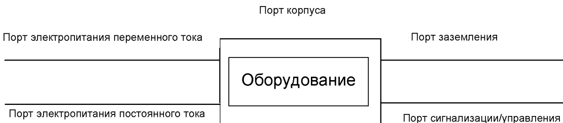
Рисунок 1 – Пример портов
