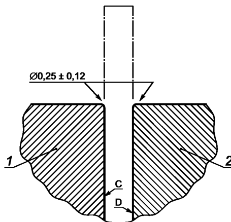
1 — неподвижная губка захватов; 2 — подвижная губка захватов
