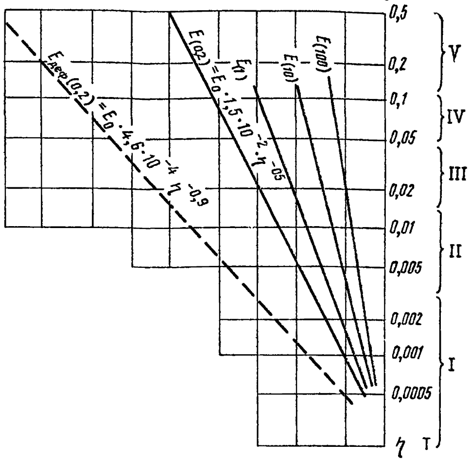
Рис. 15. Графики изменений осредненных модулей динамической упругости E и полной деформации E_{\text{деф}} для скальных пород в долях E_0 ненарушенных образцов при E=10^5 МПа и значениях трещинной пустотности 0,0005 \leq \eta \leq 0,2
