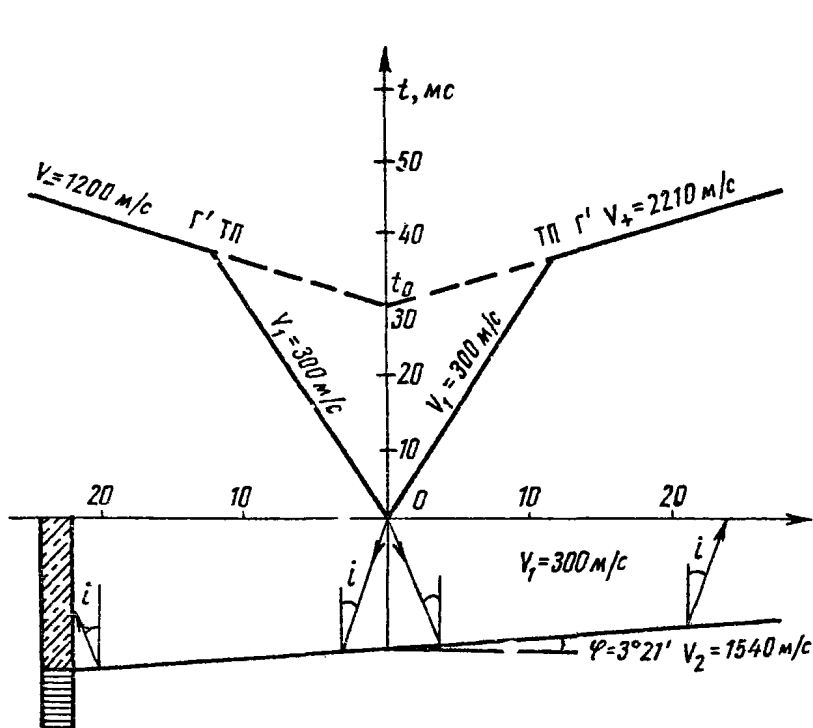
Рис. 4. Определение положения наклонной границы по годографам из одной точки
