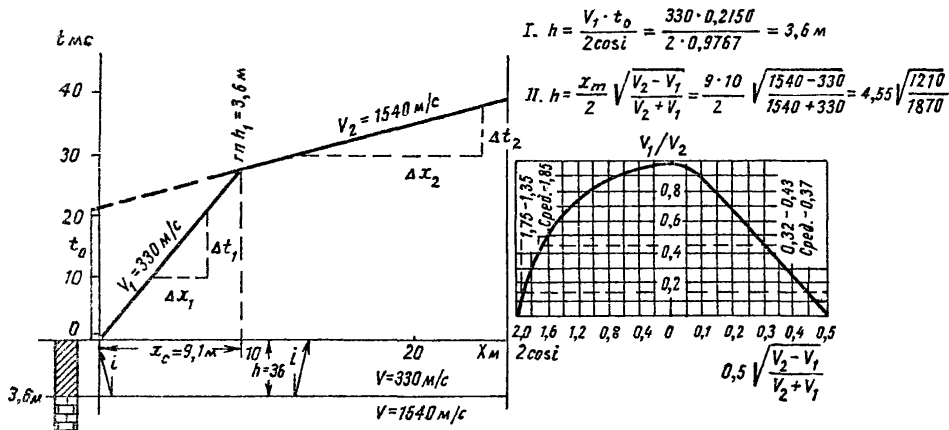
Рис. 3. Интерпретация годографа первых вступлений волны P для
