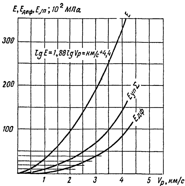
Рис. 14. Графики соотношений между скоростями распространения упругих продольных волн V_p и модулями динамической E , статической E_{\text{ст}} упругости и деформации E_{\text{дэф}} для известняков района Ингури ГЭС
