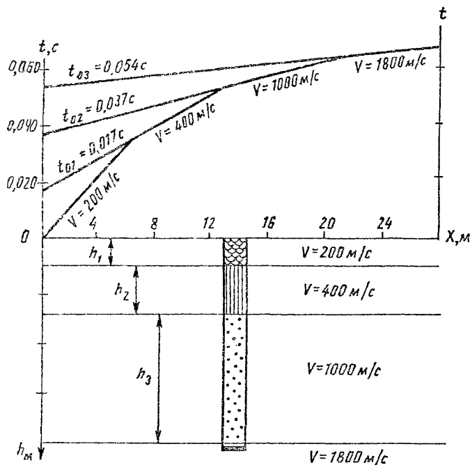
Рис. 5. Пример расчета геосейсмического разреза способом пластовых скоростей
