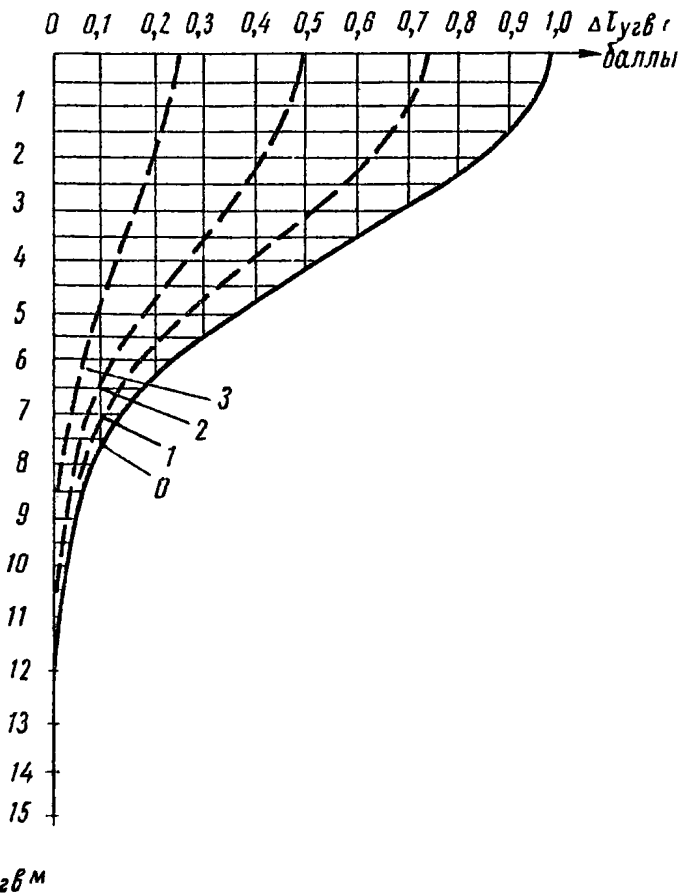
Рис. 18. Номограмма для определения приращений \Delta J_B в зависимости от глубины УГВ и подошвы обводненного слоя и скоростей V_S в них. Средние значения V_S для кривых: 0-150, 1-250, 2-500, 3-900 м/с
