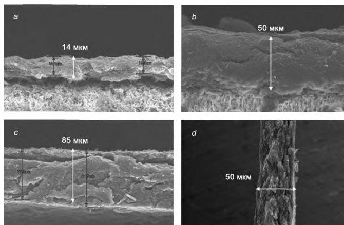
Изображения УНТ-лент, изготовленных с использованием: a — 1 мг материала из УНТ; b , d — 2 мг материала из УНТ; c — 5 мг материала из УНТ; d — изображение УНТ-ленты, демонстрирующее равномерность ее толщины
