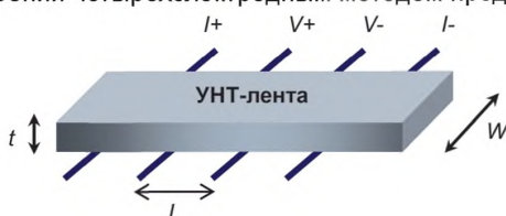
Рисунок 4 — Схема проведения измерений четырехэлектродным методом
