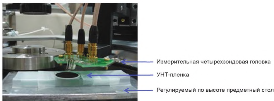
Рисунок 3 — Фотография установки с измерительной четырехзондовой головкой
