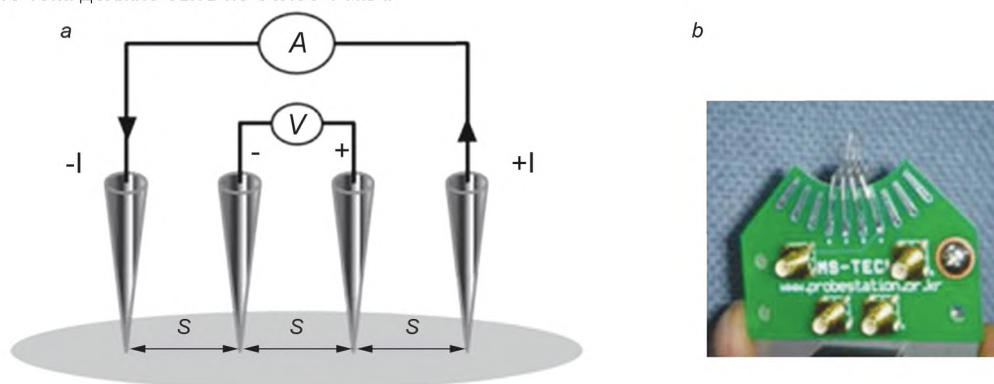
а — схема измерительной установки;
