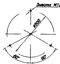
Схема расположения фундаментных болтов
