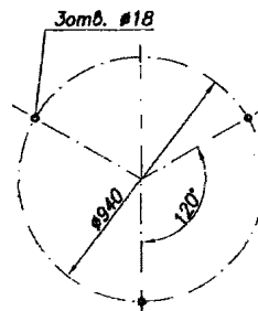
План расположения фундаментных болтов
