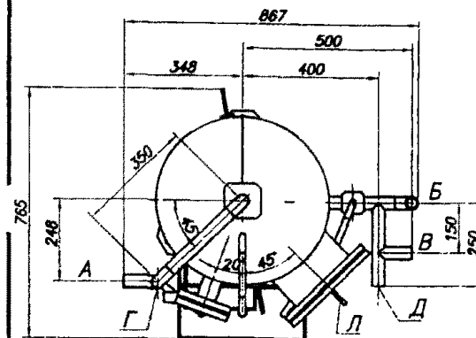
Схема расположения фундаментных болтов
