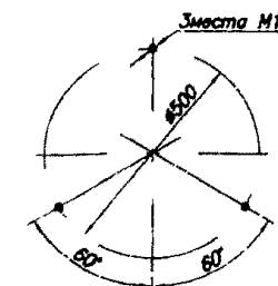
Схема расположения фундаментных болтов
