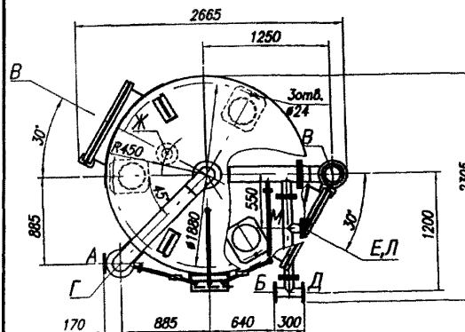
Схема расположения фундаментных болтов
