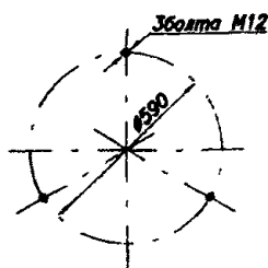
Схема расположения фундаментных болтов
