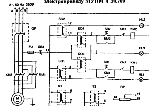
Принципиальная электрическая схема к электроприводу МУИМ и ЭХ700
