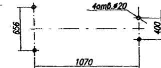
Схема расположения фундаментных болтов
