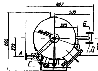
Схема расположения фрагментных болтов
