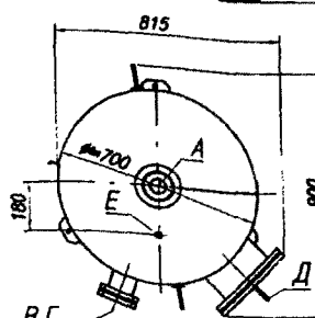
Схема расположения фундаментных болтов
