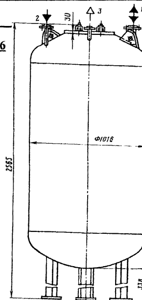
Бак напорный для вытеснения концентрированной серной кислоты БНВ-1.6: 1 — подвод и отвод кислоты, D_1 25; 2 — подача сжатого воздуха, D_2 10; 3 — спуск избытка воздуха, D_3 10
