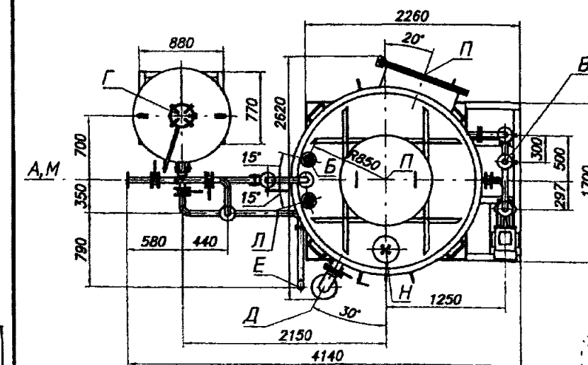
Схема расположения фундаментных болтов под рамы
