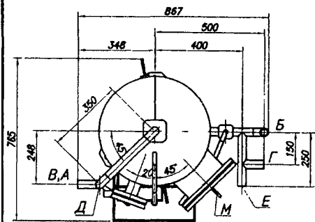
Схема расположения фундаментных болтов
