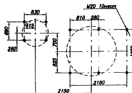
Схема расположения фундаментных болтов под рамы
