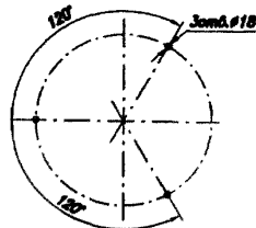
Ось вращения фундаментных болтов
