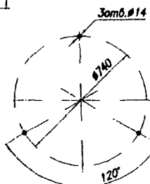
Схема расположения фундаментных болтов
