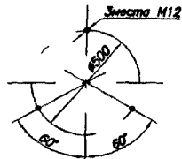
Схема расположения фрагментных болтов
