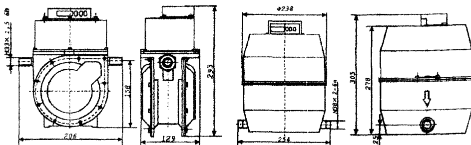
СГБ-G2,5 СГБ-G4-1
