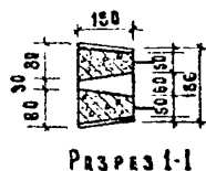
Рис.9. План и разрез железобетонных решеток марок Р2-2 и Р2-3 для комплексов крупного рогатого скота
