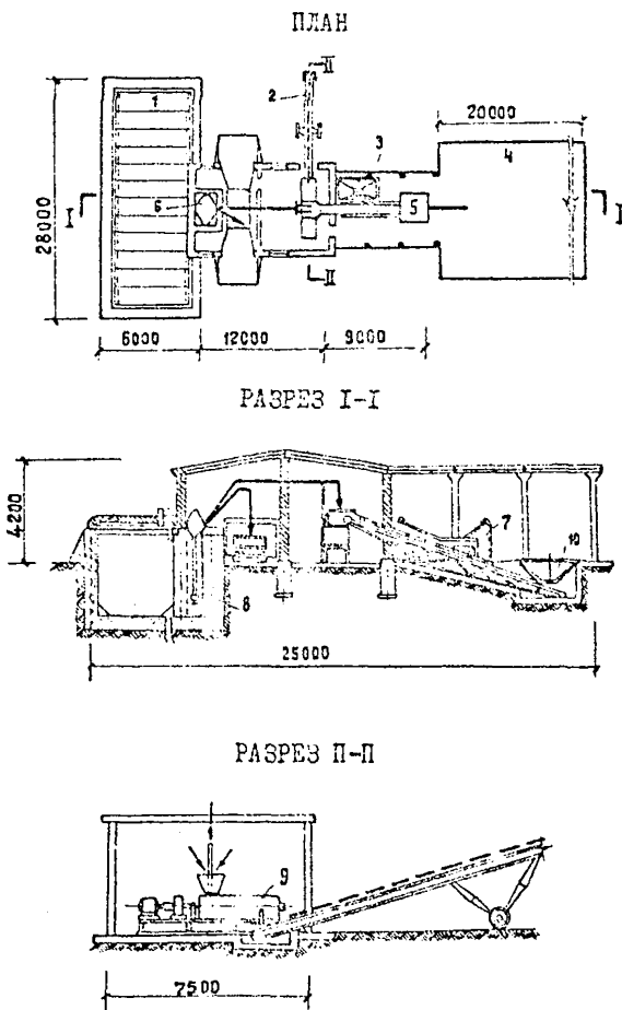
Рис.15. Компостоприготовительный цех совхоза-техникума Бологовского р-на Калининской области: I - навозохранилище; 2 - ленточный транспортер; 3 - деревянный бункер; 4 - бетонная площадка; 5 - решетка с вибратором ИВ-21; 6 - шнековый насос; 7 - переносный шнек; 8 - система рециркуляции; 9 - смеситель; 10 - бункер для торфа
