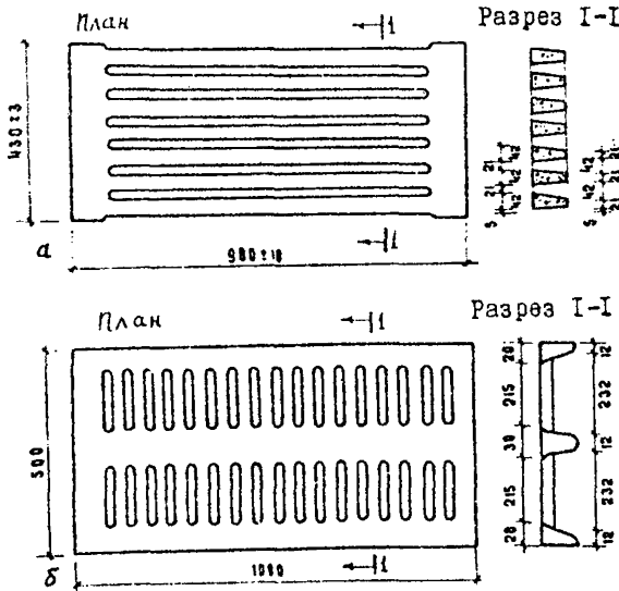
Рис. 10. План и разрез решетчатых панелей для свиноводческих комплексов: а - железобетонная панель; б - чугунная панель
