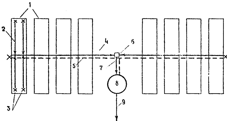
Рис.1. Основные элементы самосливной системы удаления навоза:
