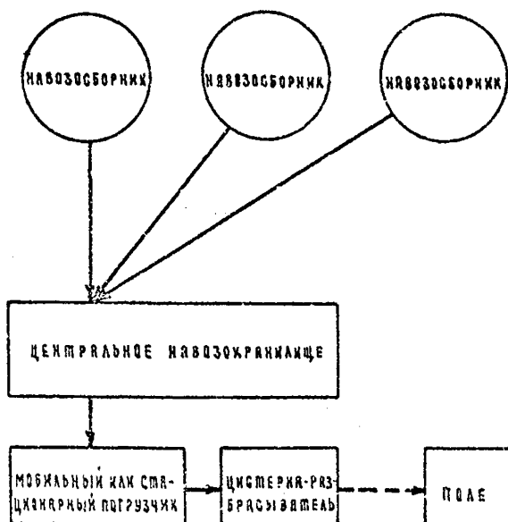
Схема 2. Доставка на поля и внесение жидкого навоза цистернами-разбрасывателями с применением мобильного погрузчика
