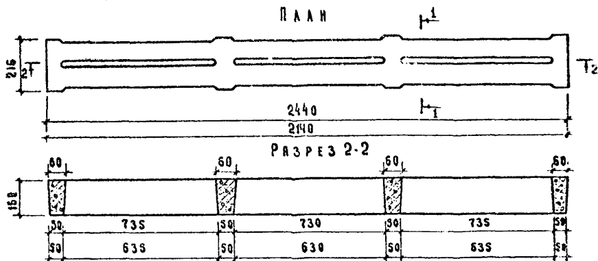
Рис.9. План и разрез железобетонных решеток марок Р2-2 и Р2-3 для комплексов крупного рогатого скота
