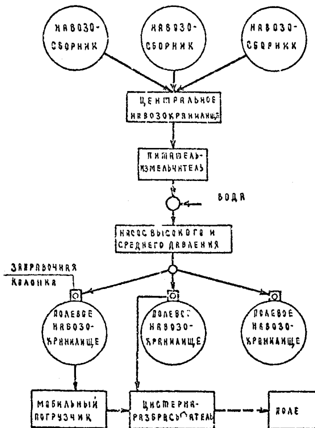
Схема 4. Транспортирование жидкого навоза по трубопроводу и внесение цистернами-разбрасывателями с самогрузкой и с применением мобильного погрузчика
