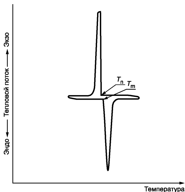
Рисунок 1 — Температуры плавления и кристаллизации чистого кристаллического материала
