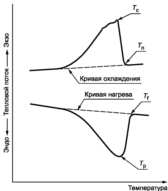
Рисунок 2 — Температуры плавления и кристаллизации полимерного материала
