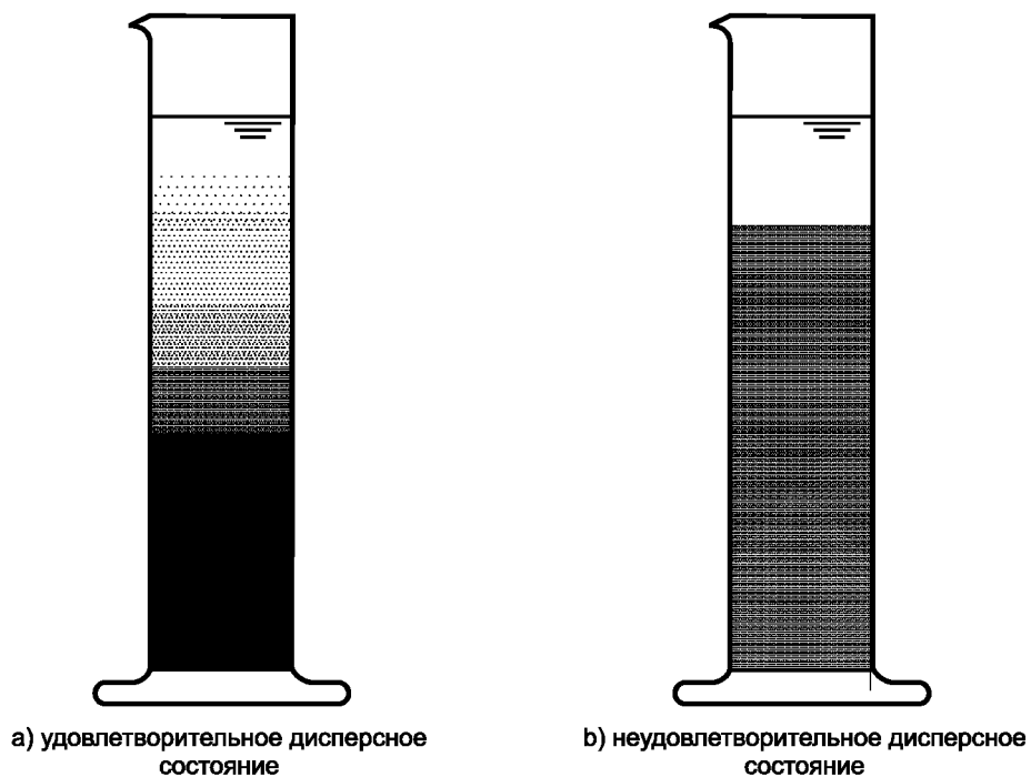
Рисунок 1 — Оценка дисперсного состояния пробы по процессу седиментации
