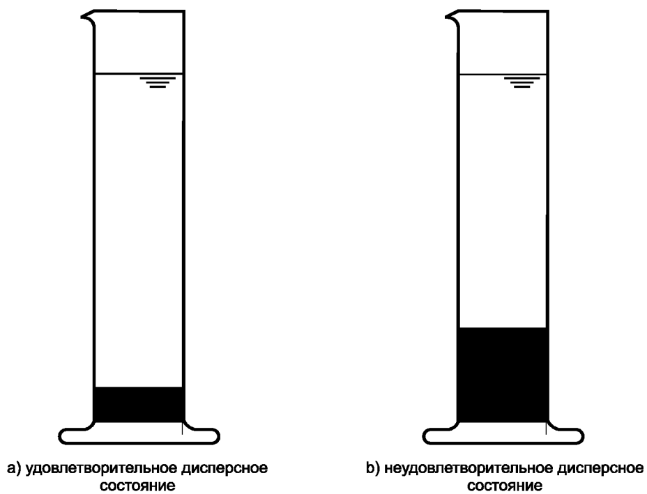
Рисунок 2 — Оценка дисперсного состояния пробы по осадку
