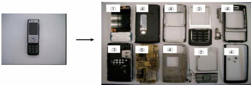
Рисунок E.3 — Частичная разборка сотового телефона (тип В) на его основные компоненты
