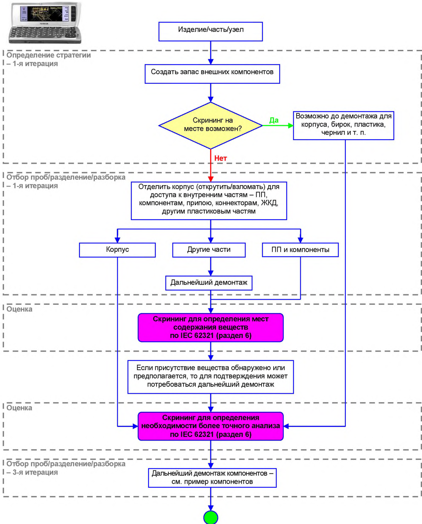
Рисунок А.5 — Отбор образцов PDA/телефона
