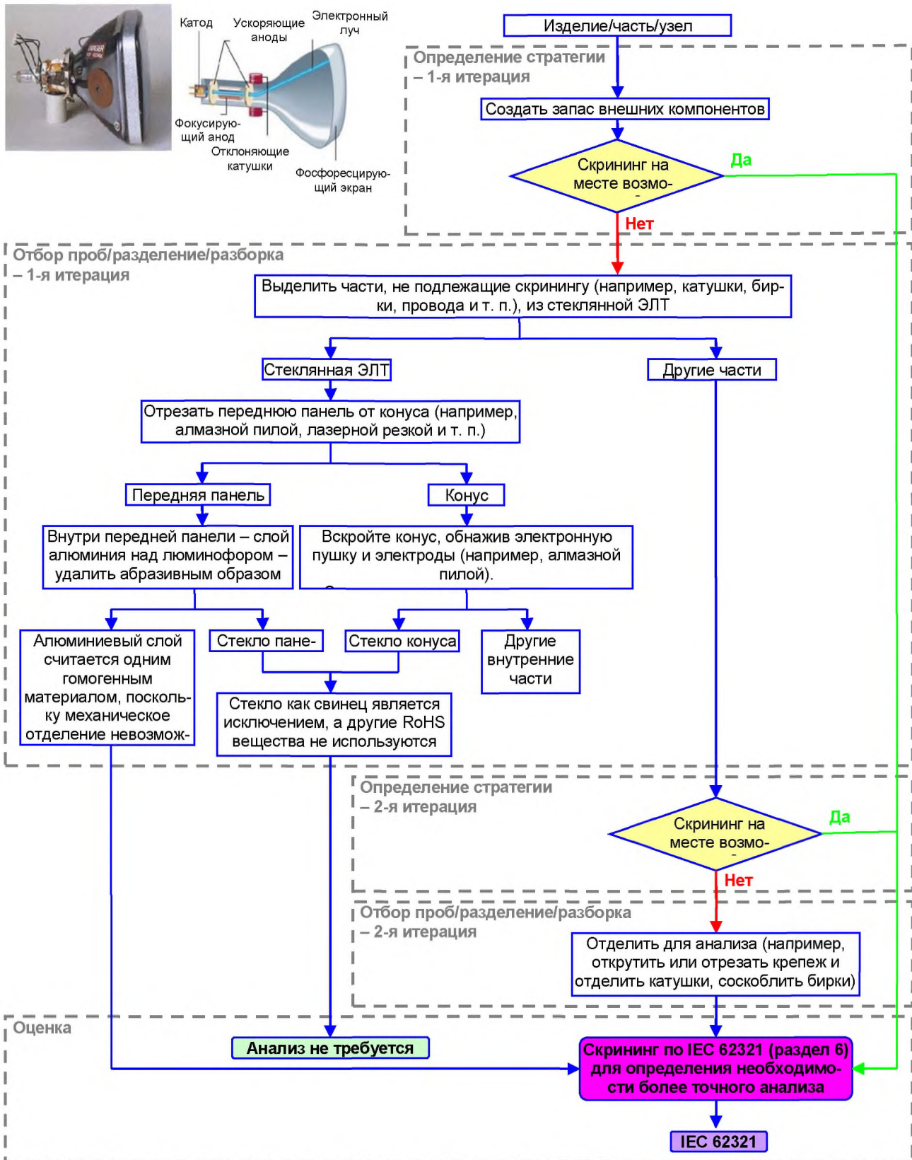
Рисунок А.3 — Отбор образцов ЭЛТ
