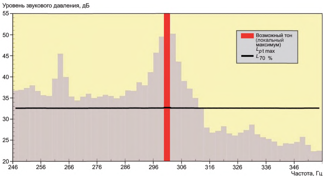
Рисунок 8 — Уровень L_{70\%} для одной критической полосы частот
