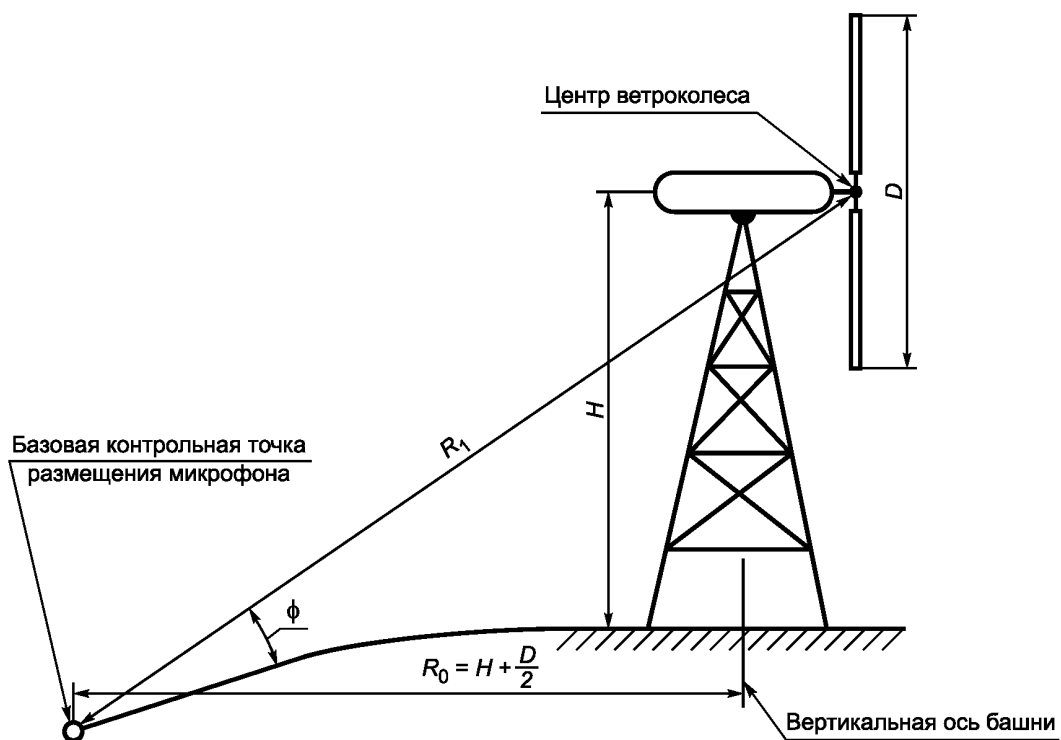
а — ветроустановка с горизонтальной осью вращения ветроколеса
