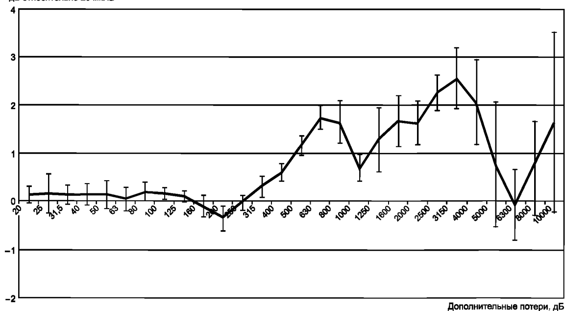
Рисунок С.1 — Пример представления данных о дополнительных потерях (поправках) при использовании дополнительного ветрозащитного экрана в виде графика (данные таблицы С.1)
