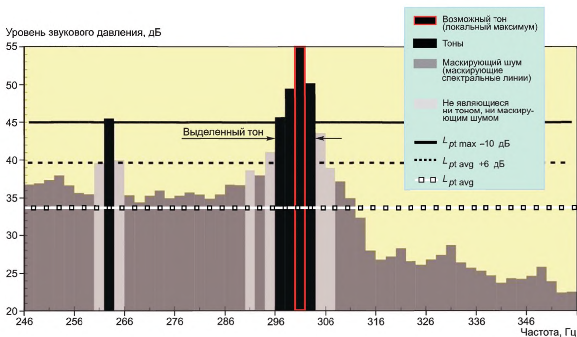
Рисунок 11 — Классификация всех спектральных линий критической полосы частот
