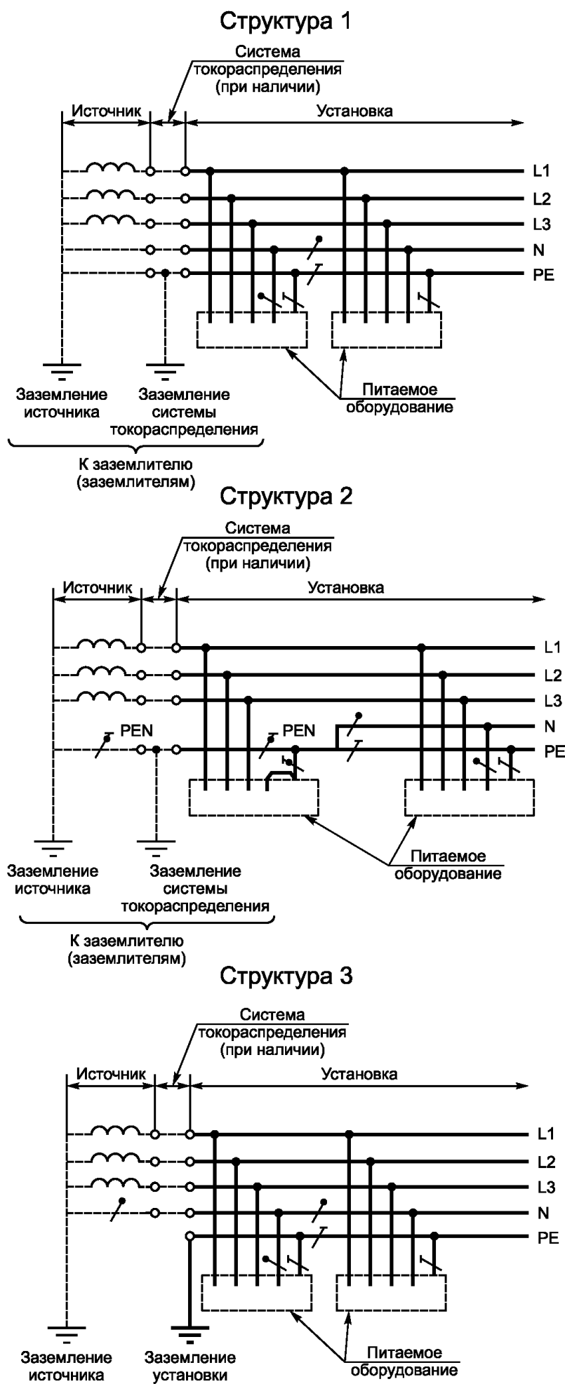
Рисунок В.1 — Стандартные системы питания от сети
