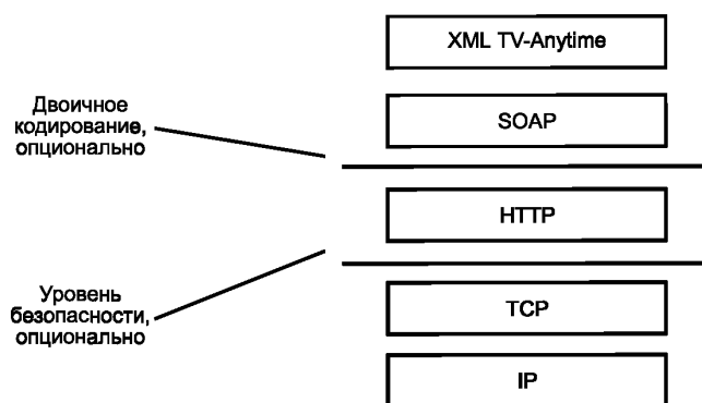
Рисунок 1 — Стек сетевых протоколов TV-Anytime
