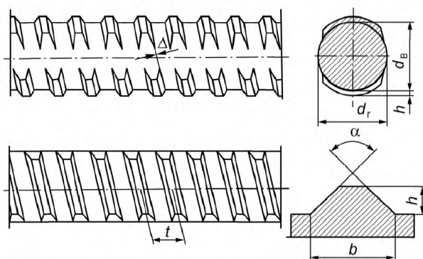
\Delta — величина отклонения винтовых выступов; d_b — максимальный диаметр винта без винтовых выступов; d_r — минимальный диаметр винта; h — высота поперечного ребра винтового выступа; t — шаг поперечного ребра; \alpha — угол наклона боковой поверхности поперечного ребра, град
