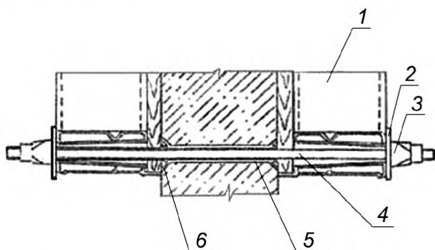
1 — щит; 2 — шайба; 3 — гайка; 4 — стяжной винт; 5 — трубка; 6 — конус
