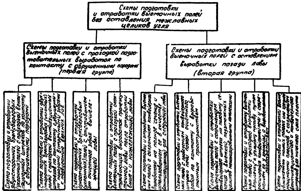
Рис. 1. 2. Классификация схем подготовки и отработки выемочных полей без оставления межлавных целлюлов угля
