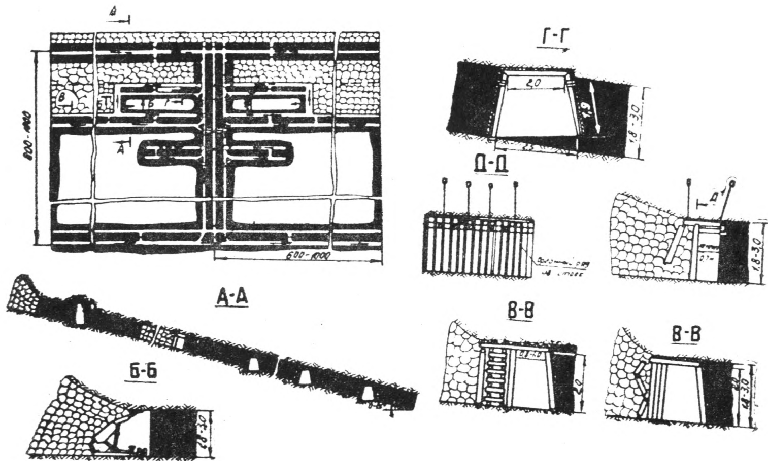
Рис. 3-10. Схема подготовки и отработки выемочных сечений и выемкой подэтажных целиков
