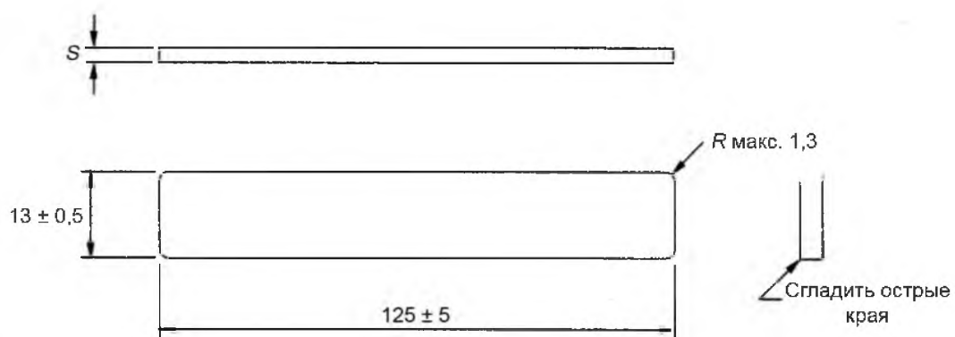
Рисунок 4 – Образец в виде полоски
