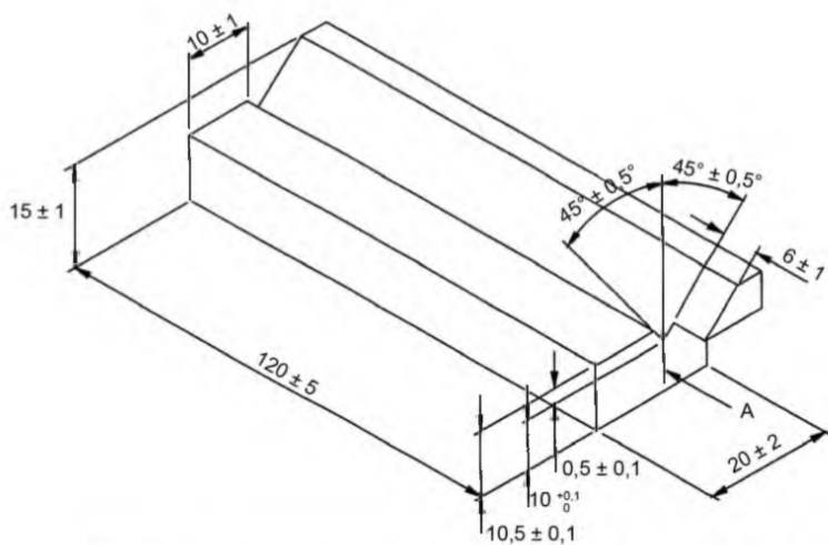
Рисунок 2 – Поддерживающая подставка для гибких образцов. Метод А
