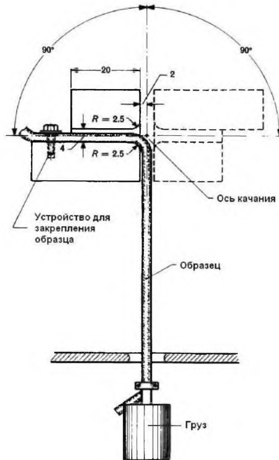
Рисунок 2 – Устройство для испытания на изгиб
