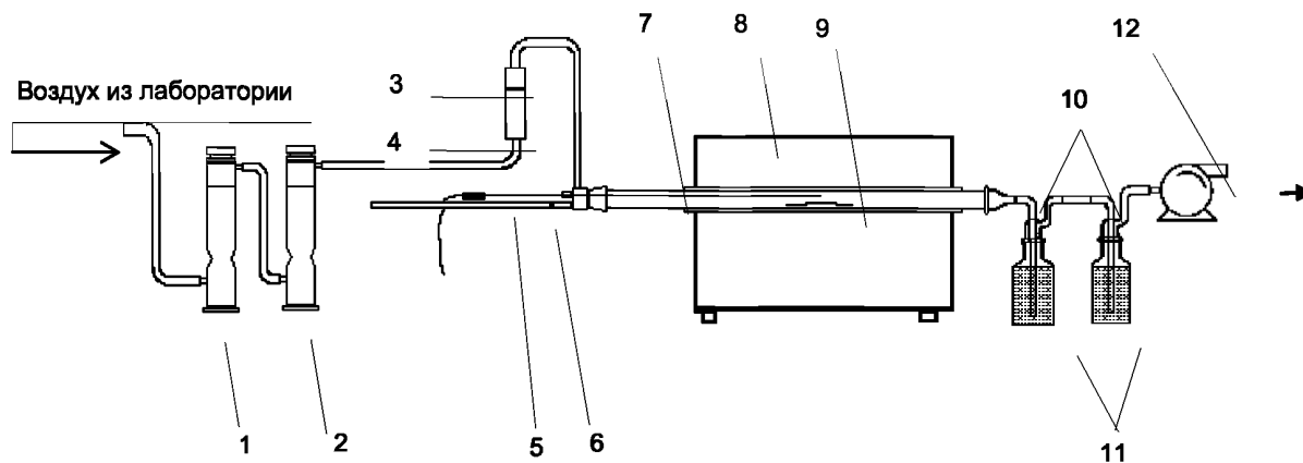
Рисунок 4 – Второй вариант установки для определения коррозионной активности газов – с подачей сжатого воздуха через редуктор с пропуском его через фильтр очистки и влагопоглотитель
