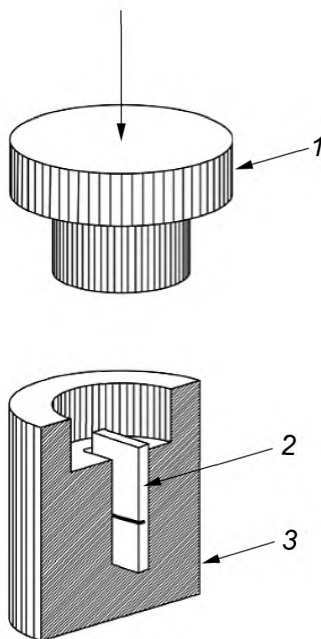
1 — нагружающий поршень; 2 — образец; 3 — корпус с пазом
