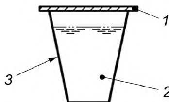
1 — крышка; 2 — бетон; 3 — емкость для проб
