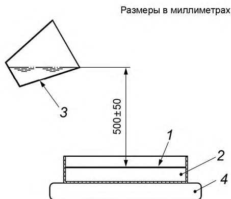
1 — сито, 2 — сборник, 3 — емкость для проб; 4 — весы
