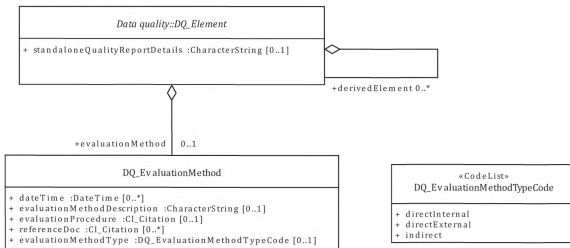
Рисунок 7 — Метод оценки качества данных
