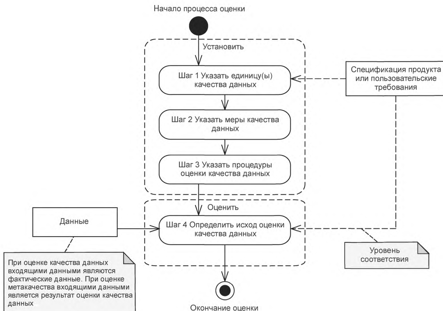
Рисунок 12 — Процесс оценки качества данных
