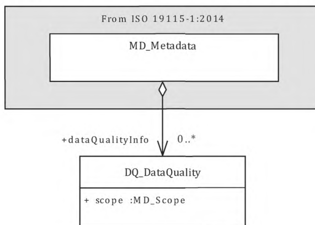
Рисунок В.2 — Информация о качестве данных
