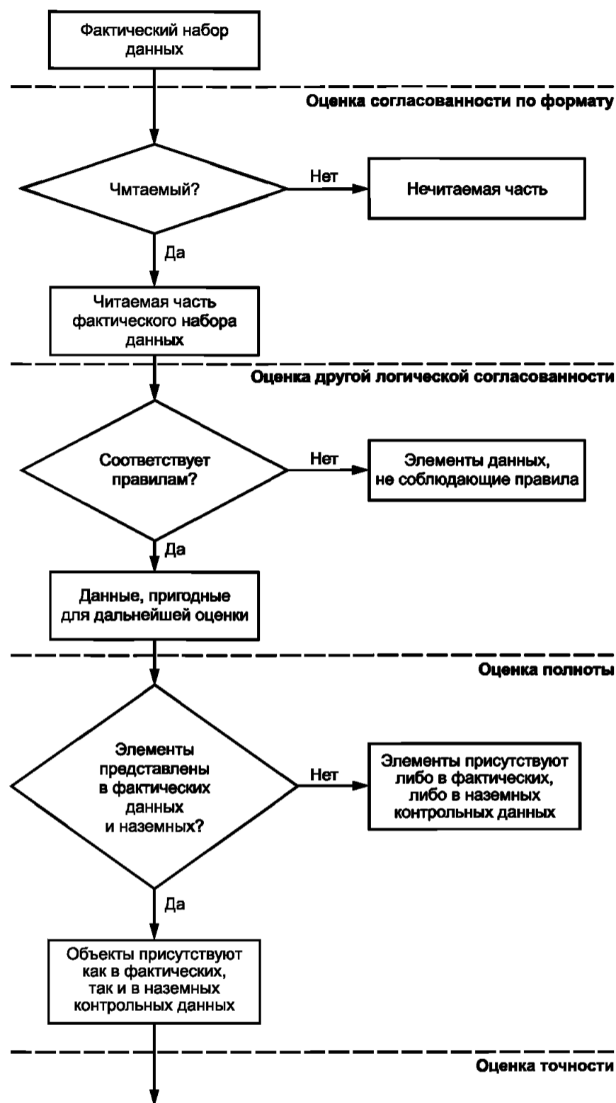
Рисунок I.1 — Порядок при оценке качества данных
