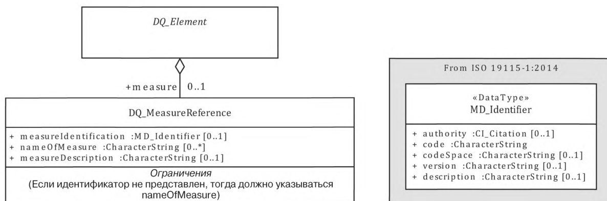
Рисунок 6 — Ссылки на меры качества данных
