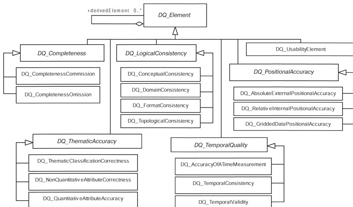
Рисунок 4 — Обзор элементов качества данных
