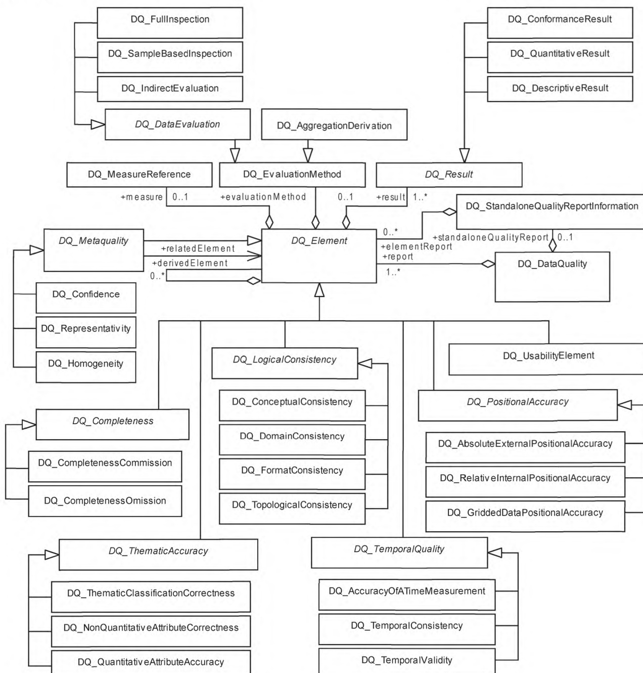
Рисунок 2 — Обзор компонентов качества данных
