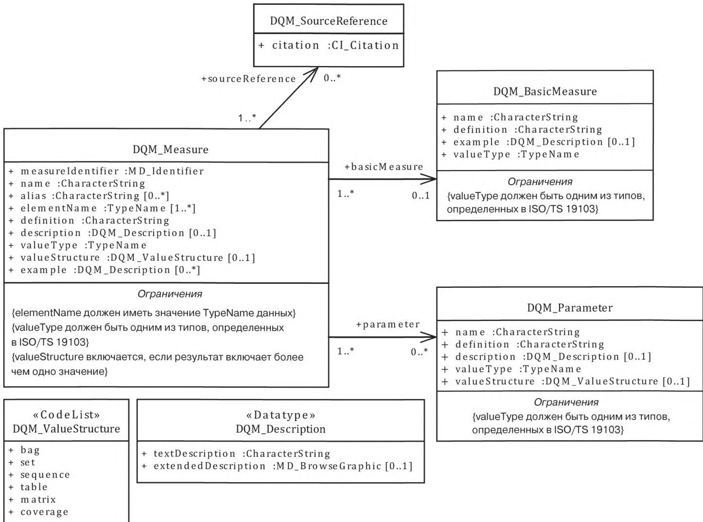
Рисунок 11 — Меры качества данных
