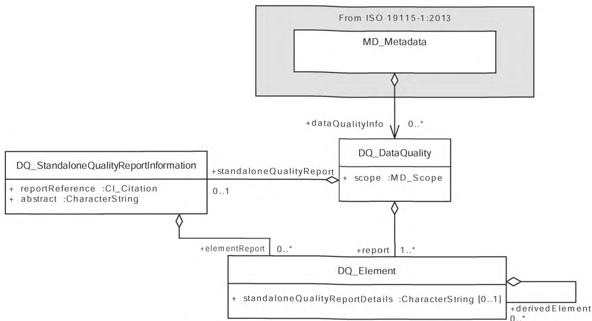
Рисунок 14 — Отчетность о качестве данных
