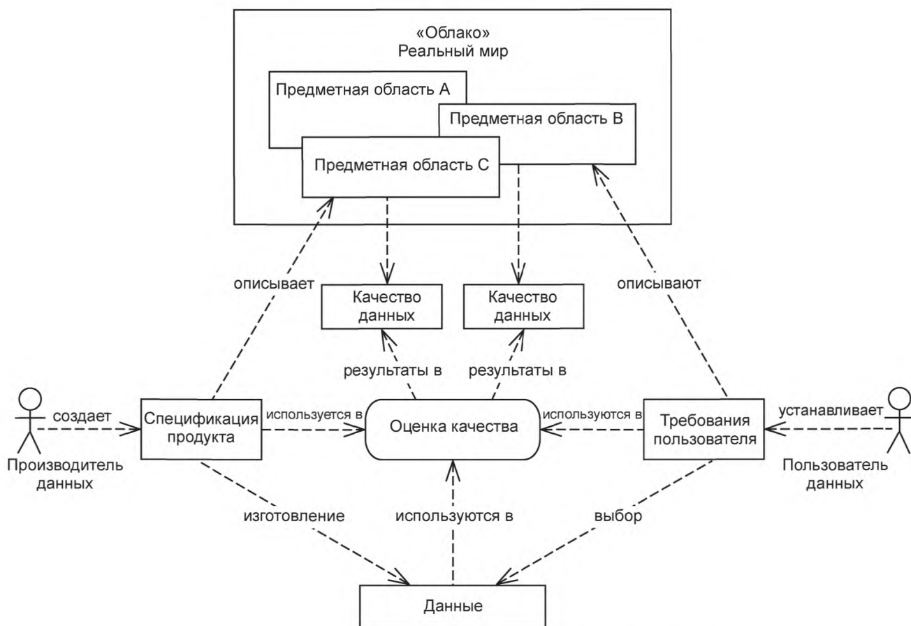
Рисунок В.1 — Концептуальные основы оценки качества данных
