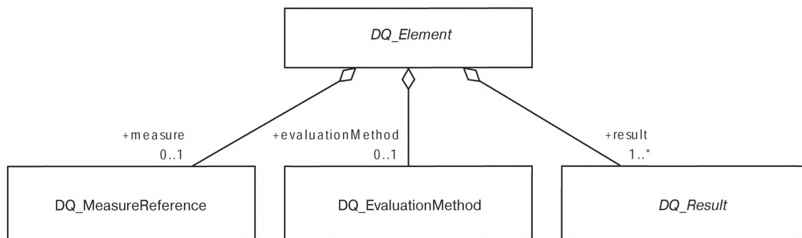
Рисунок 5 — Дескрипторы элементов качества
