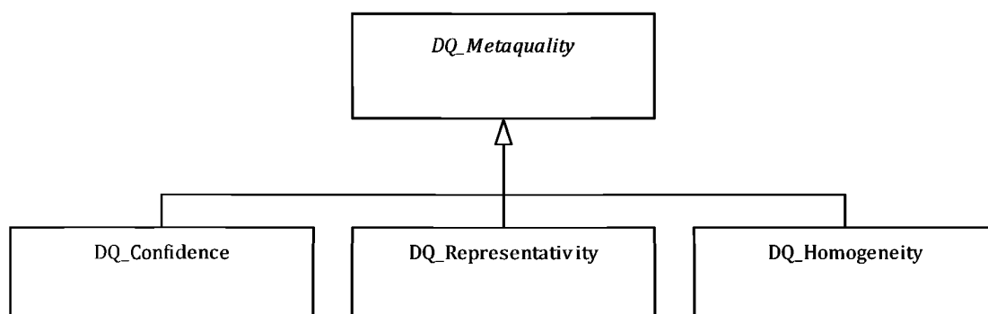
Рисунок 9 — Элементы метакачества
