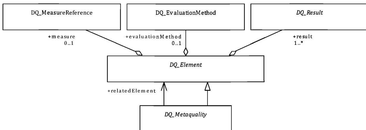
Рисунок 10 — Дескрипторы метакачества
