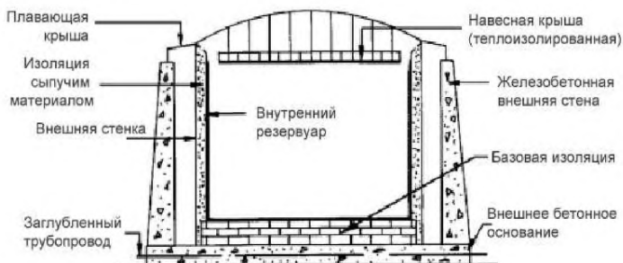
Рисунок 10 – Резервуар с двойной стенкой
