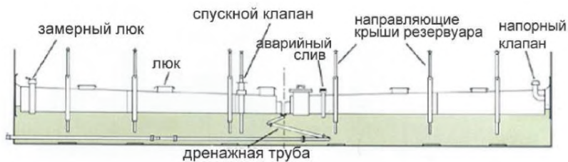
Рисунок 3 – Пример типичной двойной плавающей понтонной крыши
