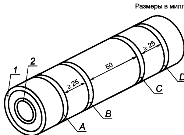
Рисунок D.1 — Подготовка образцов для измерения удельного объемного электрического сопротивления экранов по жиле и по изоляции
