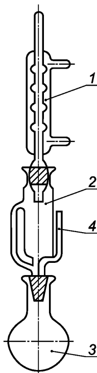
1 — холодильник; 2 — экстрактор; 3 — экстракционная колба; 4 — сифонная трубка
