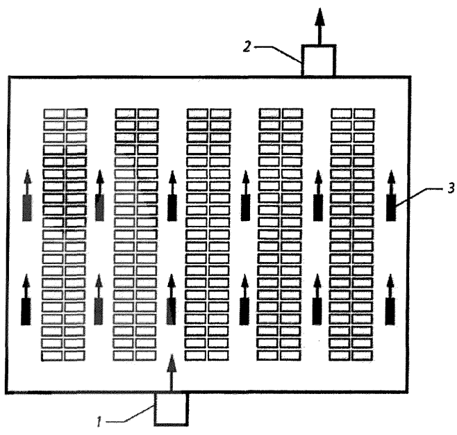
1 – система приточной вентиляции; 2 – система вытяжной вентиляции; 3 – струйный вентилятор
