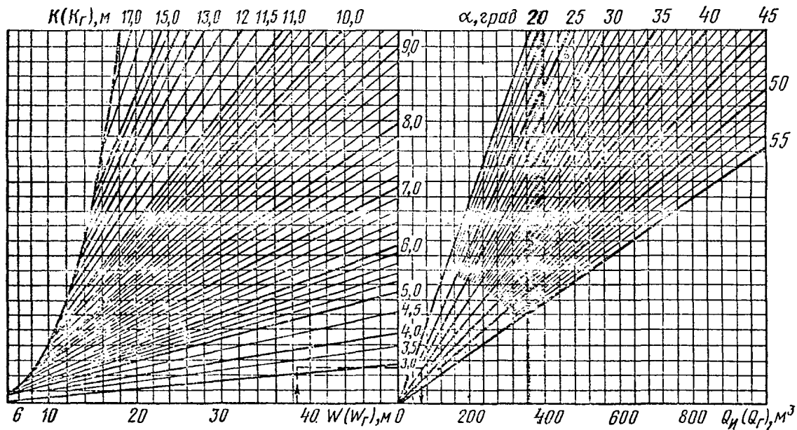
Рис. 2. Номограмма для определения объемов буртов (до 1000 м 3 ) на прямоугольных в плане площадках (отсеках).
