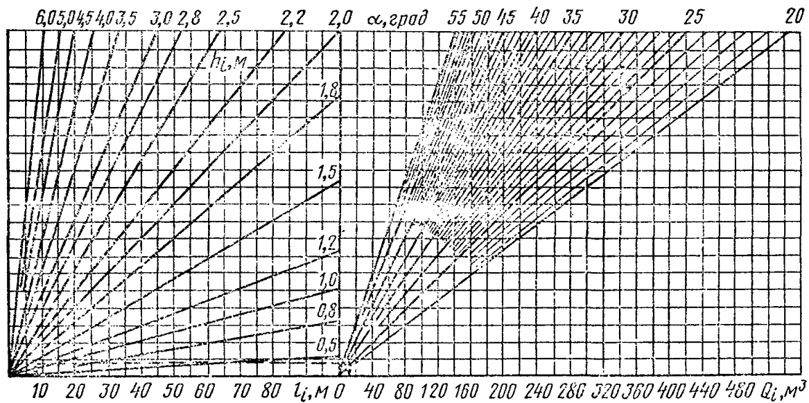
Рис. 4. Номограмма для определения отсекаемых подпорными стенами частей буртов при различных схемах расположения подпорных стен (объемы частей буртов до 560 \text{ м}^3 ):
