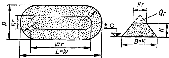
Рис. 6. Параметры бурта без подпорных стен.
