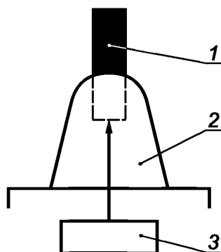
1 — образец; 2 — приспособление для испытания; 3 — датчик деформации
