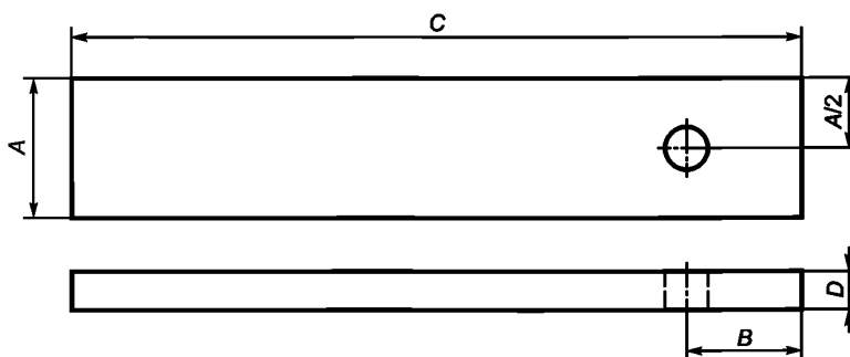
Рисунок 4 — Образец для испытаний
