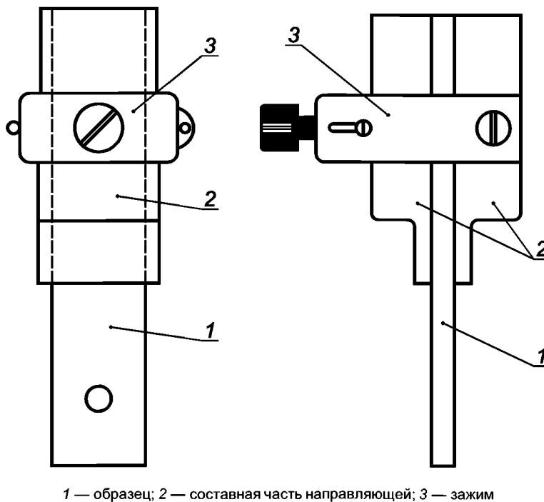
Рисунок 3 — Общий вид направляющей
