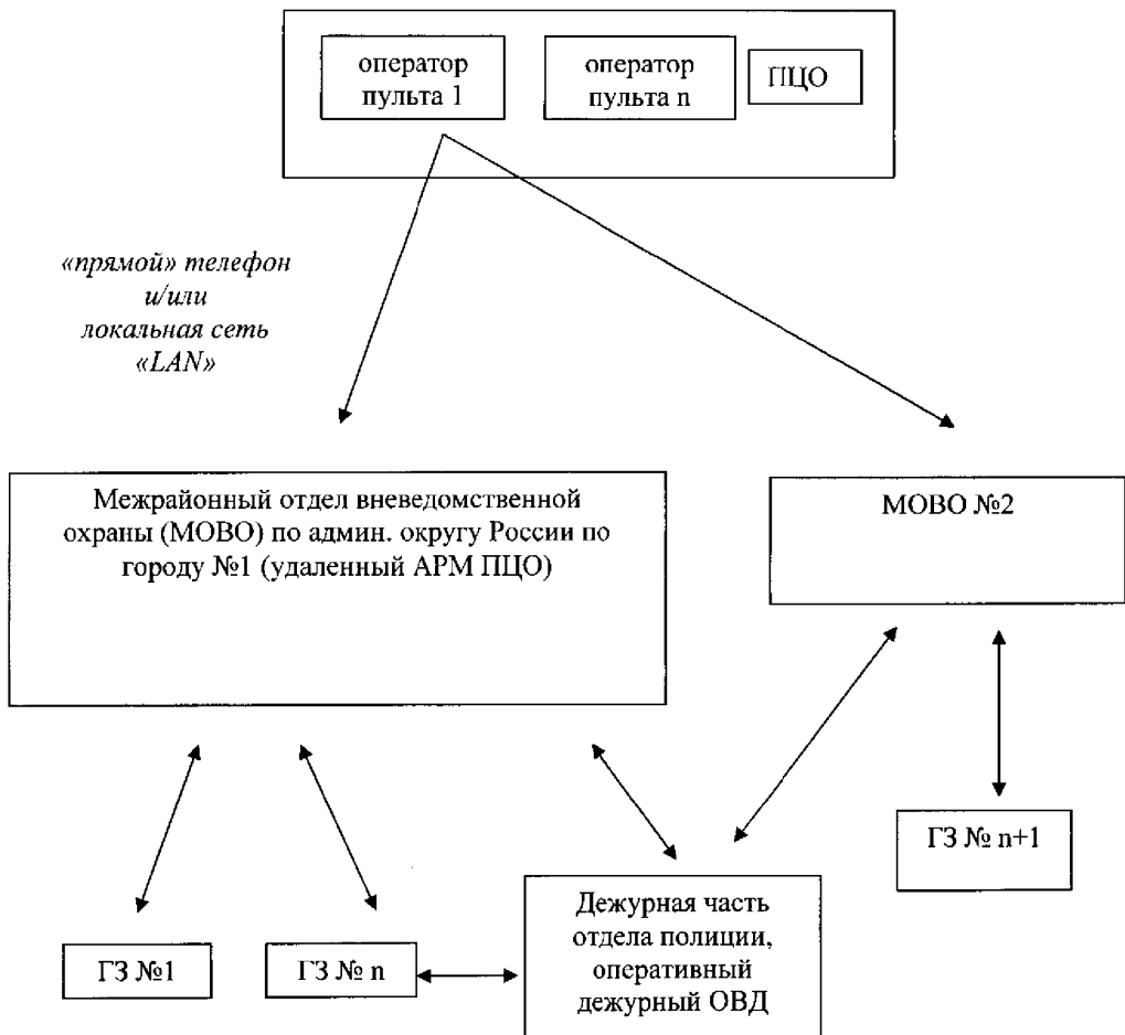
Рисунок 3 -ПЦО без дежурного, схема взаимодействия (средний город)
