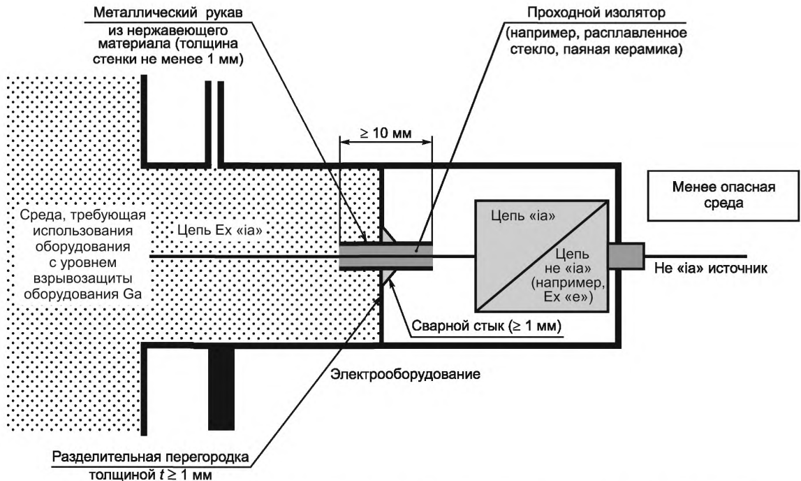
Рисунок 1 — Пример газонепроницаемой разделительной перегородки с проходным изолятором
