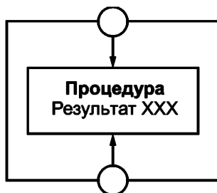
Рисунок 3 — Процедурное правило
