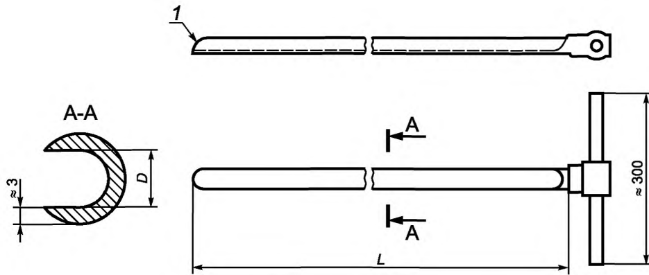
1 — острая кромка; D — внутренний диаметр; L — длина
