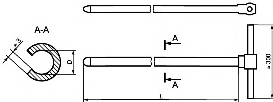
D — внутренний диаметр; L — длина
