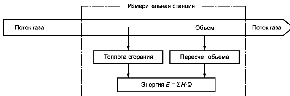
Рисунок 6 — Локальное онлайн измерение теплоты сгорания
