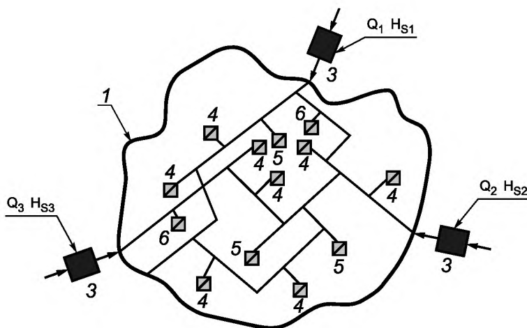
1 — зона газопотребления; 3—6 — пункты приема-передачи
