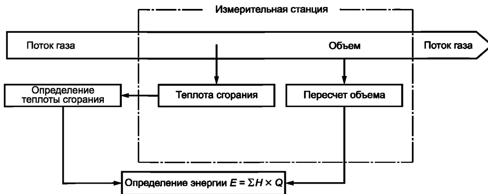
Рисунок 7 — Локальное офлайн определение теплоты сгорания
