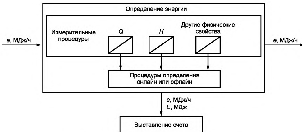
Рисунок 2 — Схема определения энергии косвенным методом
