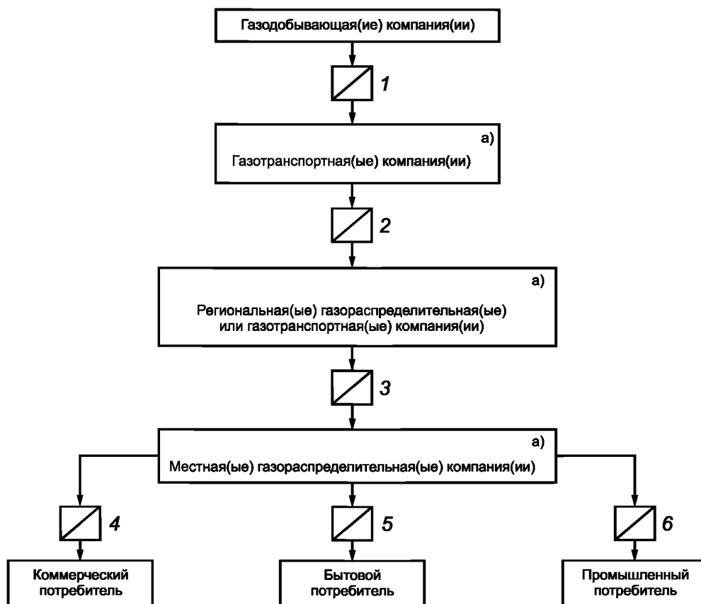
1—6 — пункты приема-передачи; а) при наличии компании
