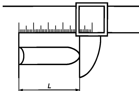
Рисунок 2 — Измерение штангенциркулем длины пеллеты между средней точкой выпуклого конца пеллеты и вогнутым поперечным сечением пеллеты
