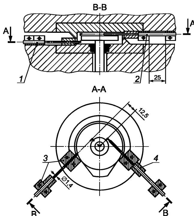
1 — удаленный измерительный зонд; 2 — вставляемый измерительный зонд; 3 — стопы, присоединенные к аппарату; 4 — стопор, присоединенный к измерительному зонду
