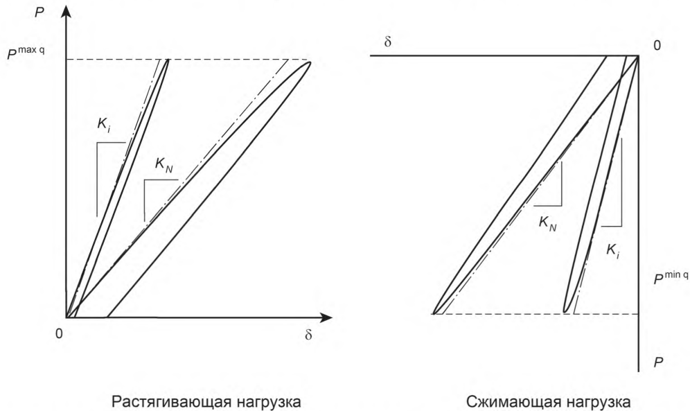
Растягивающая нагрузка
