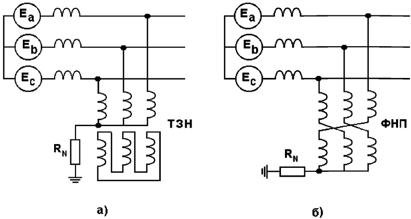
Рисунок 8.1 – Схемы включения резисторов в сети 35 кВ: а) в нейтраль обмотки высокого напряжения со схемой соединения обмоток Y0/\Delta ; б) в нейтраль фильтра нулевой последовательности
