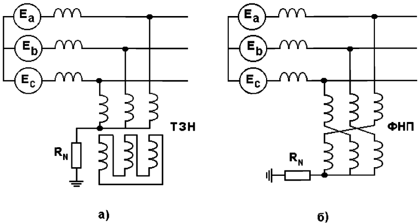
Рисунок 7.1 – Схемы подключения резистора к нейтрали сети
