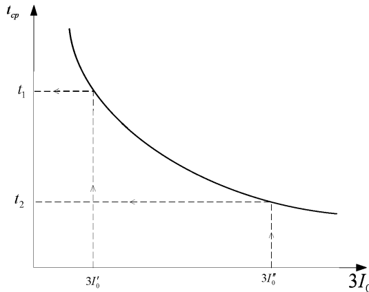
Рисунок В.4 – Обратная-зависимая характеристика выдержки времени t_{C3} защиты от тока ОЗЗ
